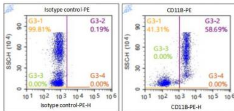
图. 人外周血染色左图为Mouse IgG1 Isotype control,PE, 右图为 Anti-Human CD11b,PE (Clone: LT11) (F11011b02/3) 的结果。以淋巴细胞、粒细胞和单核细胞设门进行分析。
